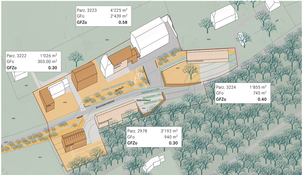
Bebauungsvariante M, f. M.
