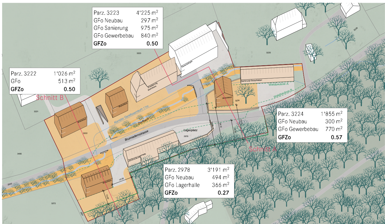
Bebauungskonzept, freier Massstab (f. M.)
