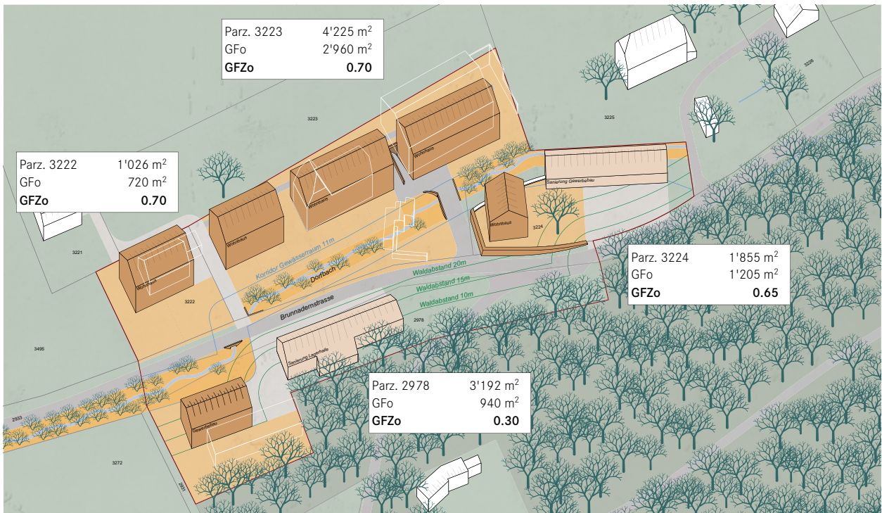
Bebauungsvariante L, f. M.
